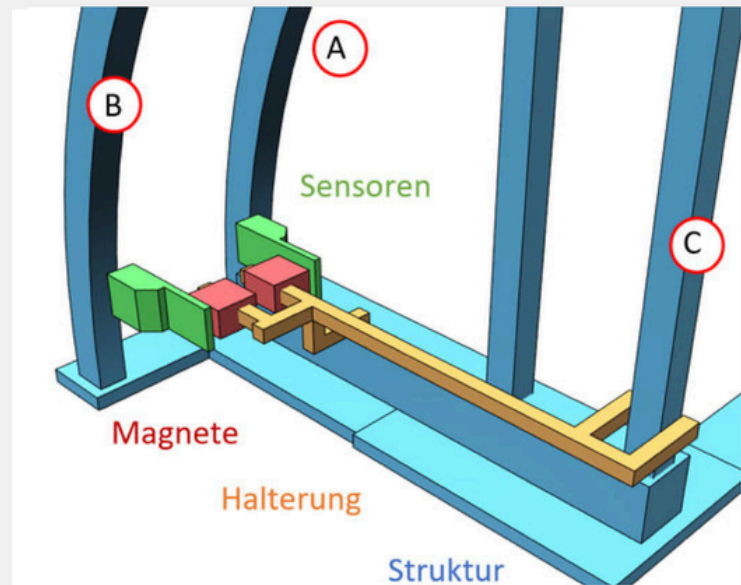
Schematischer Messaufbau mit den Sensoren an den zu messenden Stützen A und B sowie der Halterung zum Referenzpunkt C.
