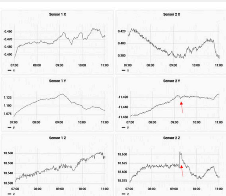
Messwerte von zwei Sensoren in der X, Y und Z-Achse.
